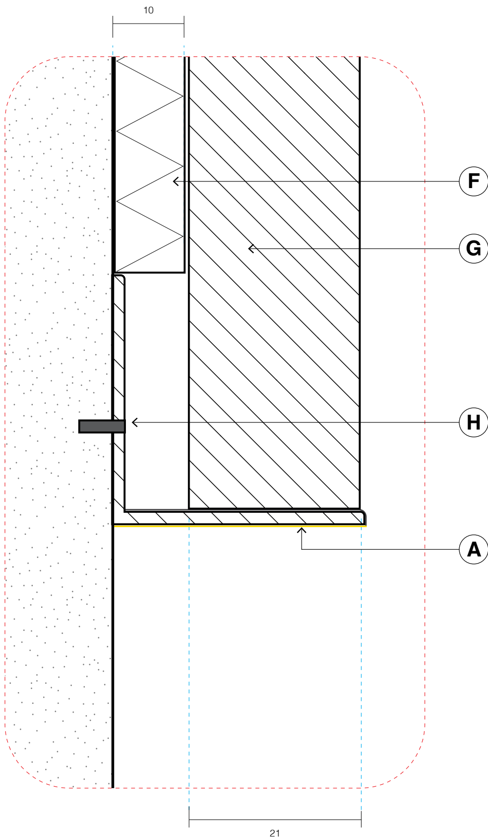
02 Detail Bottom edge Scale 2:1
