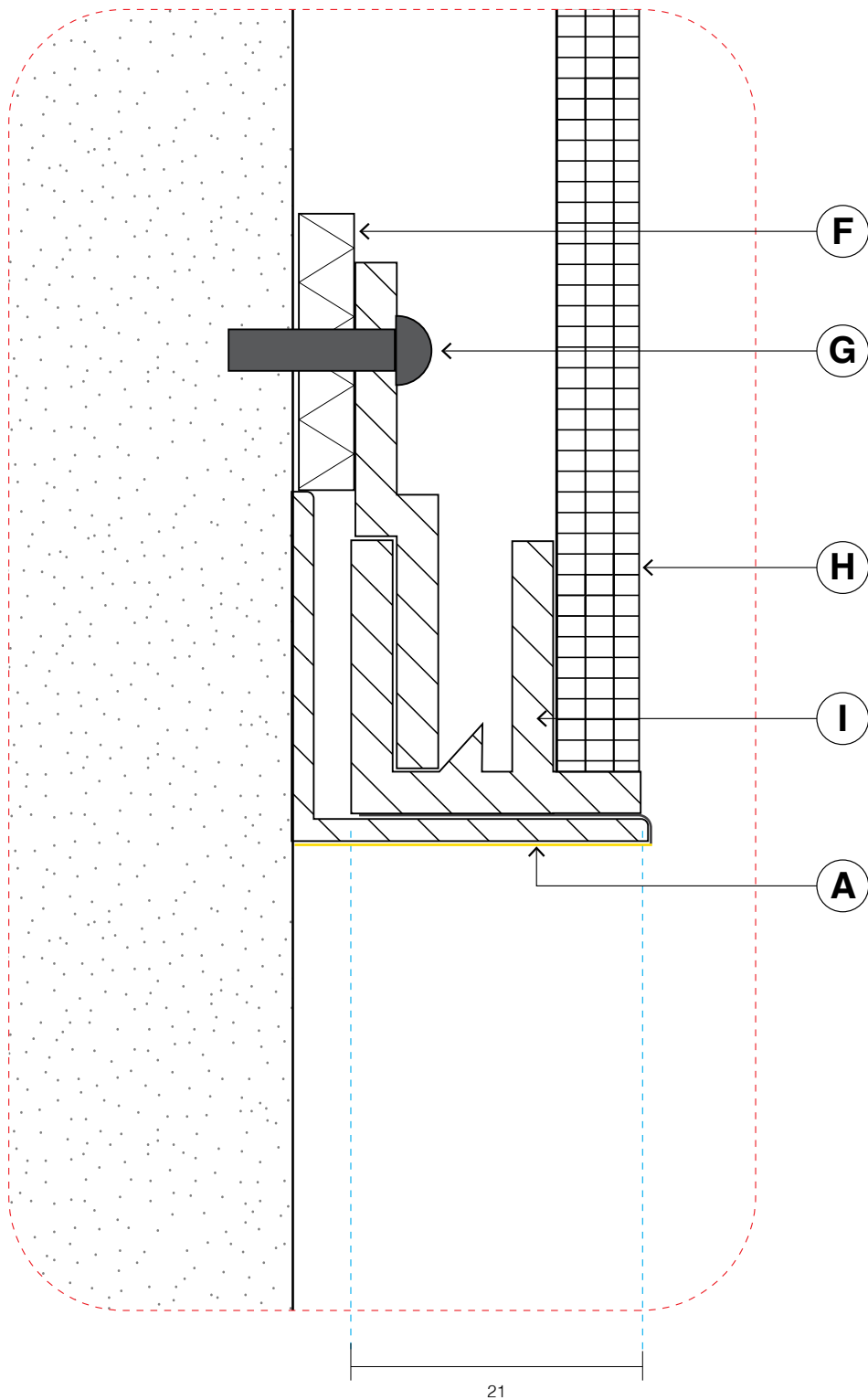
02 Detail Bottom edge Scale 2:1
