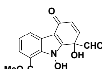
Coproverdine
