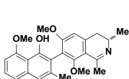
Ancistrotanzanine A
